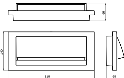
Maße ZAW Dimensions ZAW
